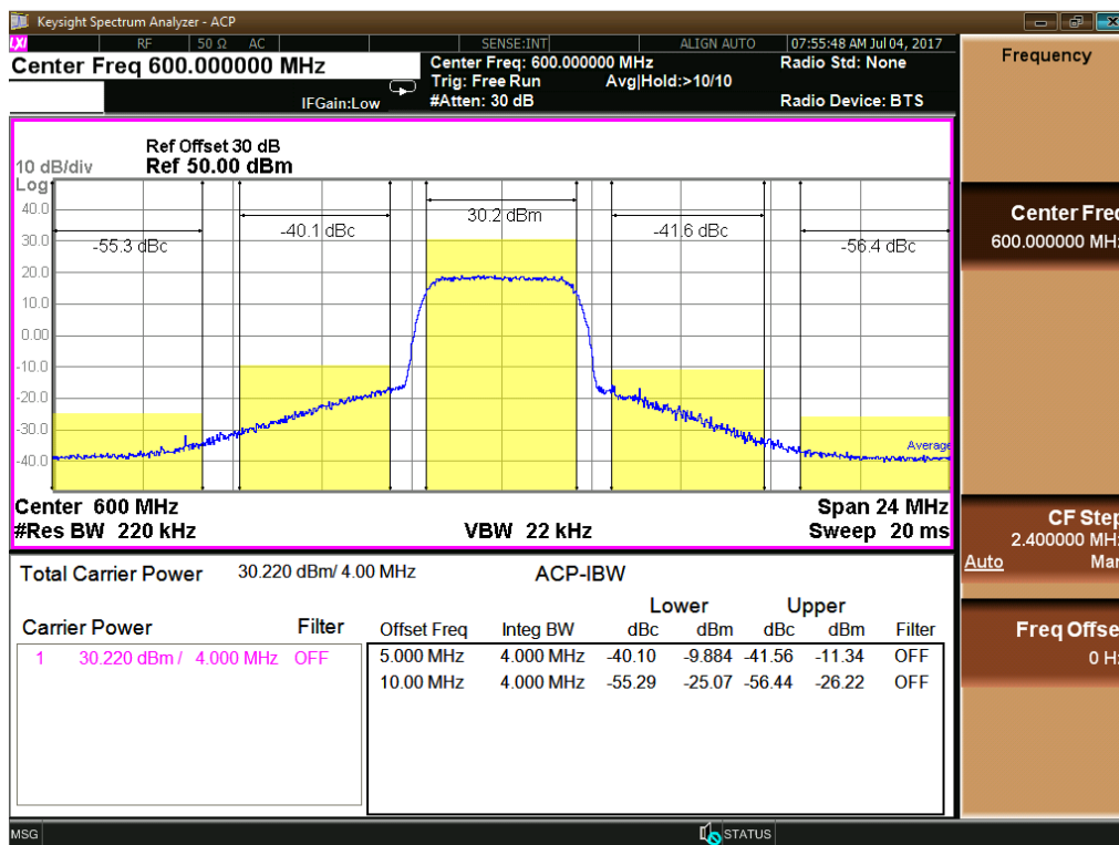
Pout @WCDMA 600MHz PAR=9.9dB
