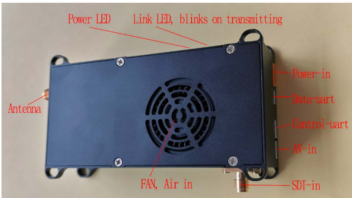
ST210-SDI
